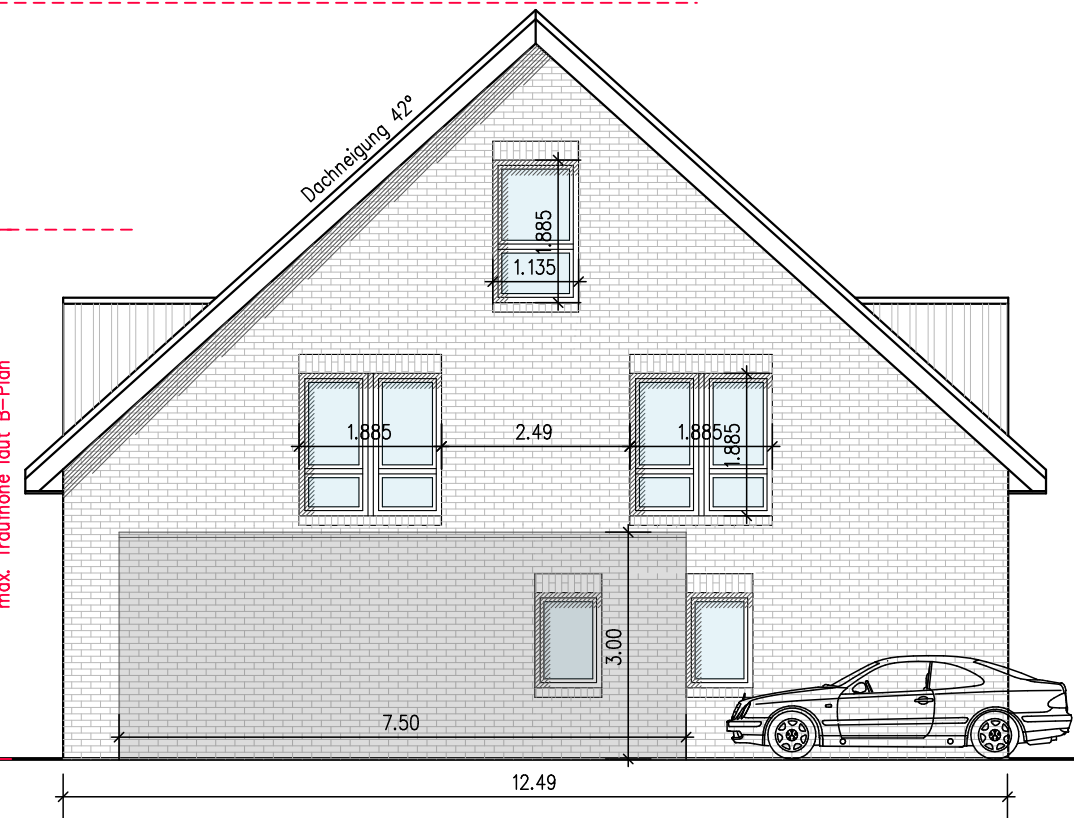
Nord-Westansicht Grundstück_7
